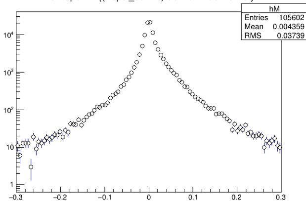
PsProperDL {(NJpsi_ee==1) && Pt>4 && Pt < 5 }
