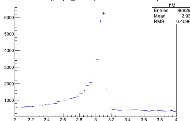
Mass {(NJpsi_ee==1) && Pt>5 && Pt < 7 }
