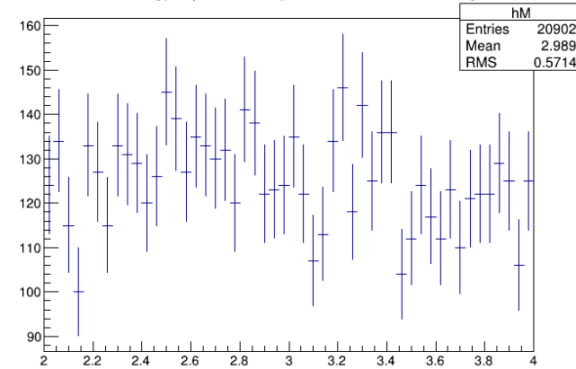
Mass {(NJpsi_ee!=1) && Pt>7 && Pt<10 }
