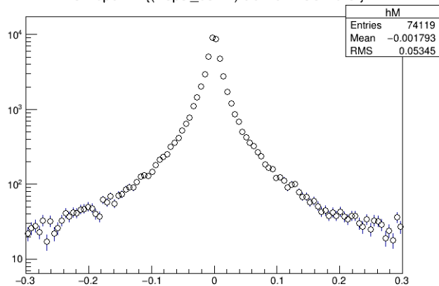
PsProperDL {(NJpsi_ee!=1) && Pt>4 && Pt<5 }
