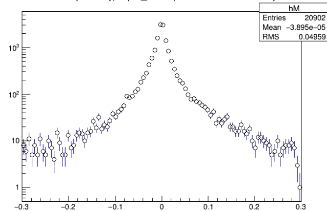
PsProperDL {(NJpsi_ee!=1) && Pt>7 && Pt<10 }
