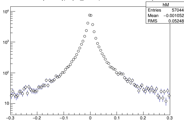
PsProperDL {(NJpsi_ee!=1) && Pt>5 && Pt<7 }
