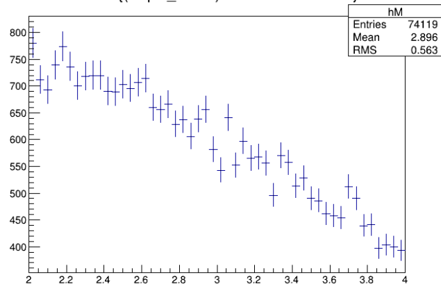
Mass {(NJpsi_ee!=1) && Pt>4 && Pt<5 }
